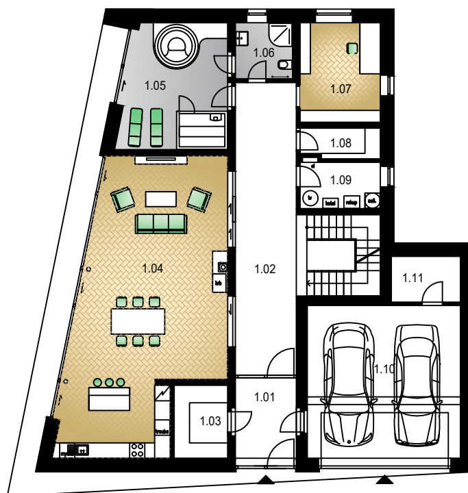
PŮDORYS 1.NP, 1:200
